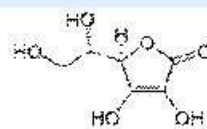
Structuur van L-ascorbinezuur
